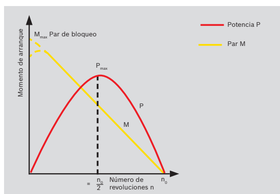
Fig. 1 Curvas características de un motor neumático
