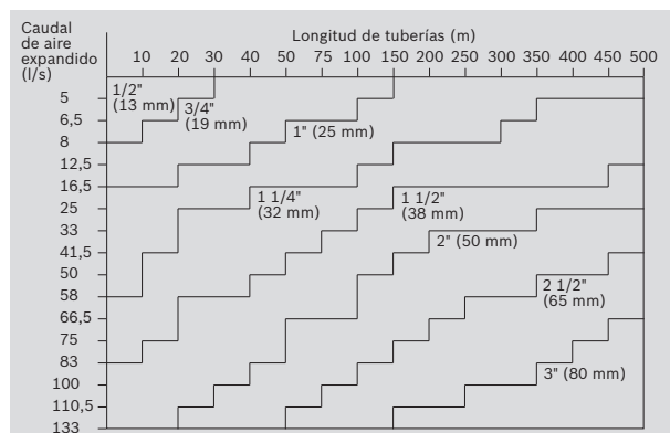
Fig. 5 Cálculo del tamaño de tubería
