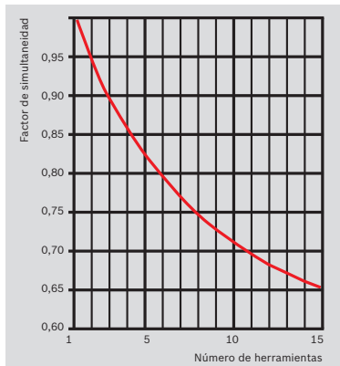
Fig. 3 Factor de simultaneidad
