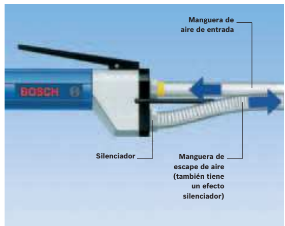
Fig. 7 La manguera de escape de aire protege al usuario, el medio ambiente y la pieza de trabajo
