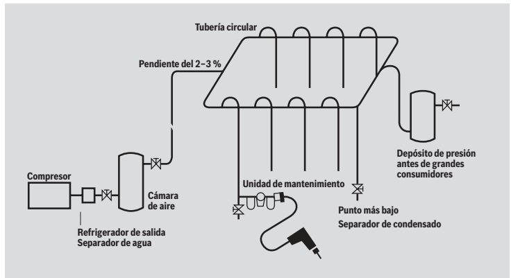
Fig. 4 Esquema de una instalación de aire comprimido
