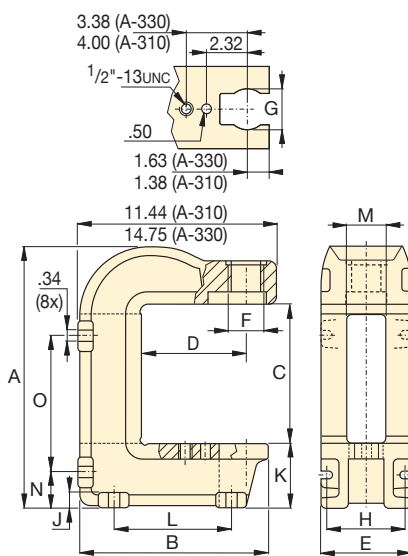
Prensas de husillo, modelos A-310, A-330
