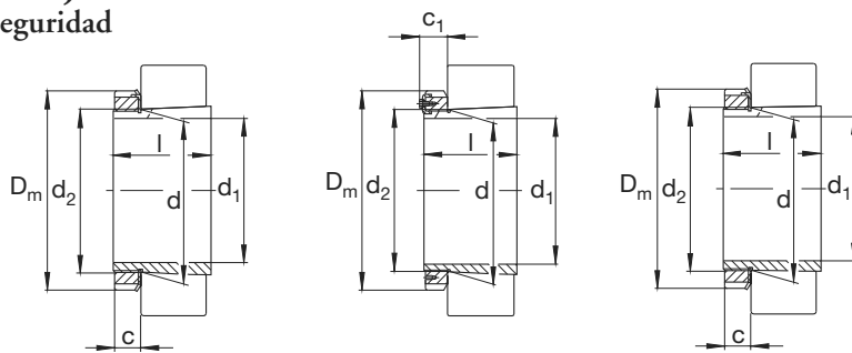
Cono 1:12 Chapa de seguridad MB, MBL
