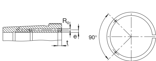
Manguito de desmontaje hidráulico (sufijo H)
