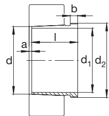
AH240, AH241 Cono 1:30
