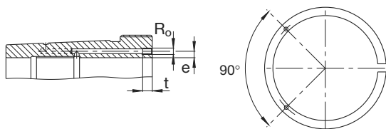
Manguito de desmontaje hidráulico (sufijo H)
