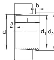
AH240, AH241 Cono 1:30
