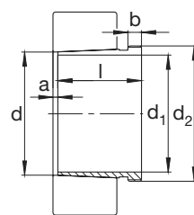
AH240, AH241 Conol 1:30
