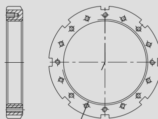
HM30H, HM31H Agujeros roscados para tornillos de montaje (bajo demanda)
