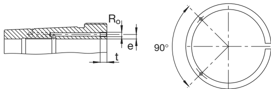
Manguito de desmontaje hidráulico (sufijo H)
