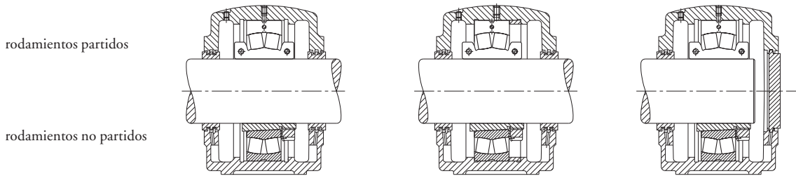
Soporte: Rodamiento libre SDAF5 Rodamiento fijo SDAF5 Rodamiento libre SDAF5
