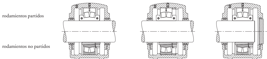
Soporte: Rodamiento libre SAF5 Rodamiento fijo SAF5 Rodamiento libre SAF5
