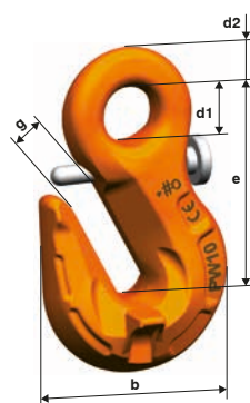
PSW Gancho paralelo con fiador
