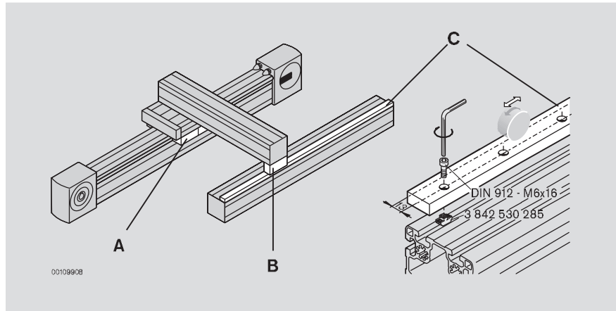
Cojinete de sustentación LF20
