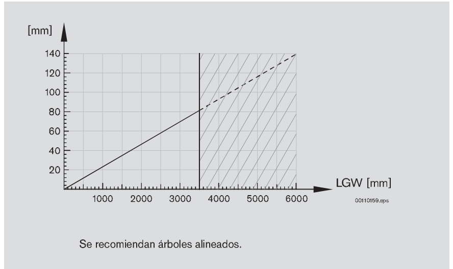
Diagrama 4: Desplazamiento lateral
