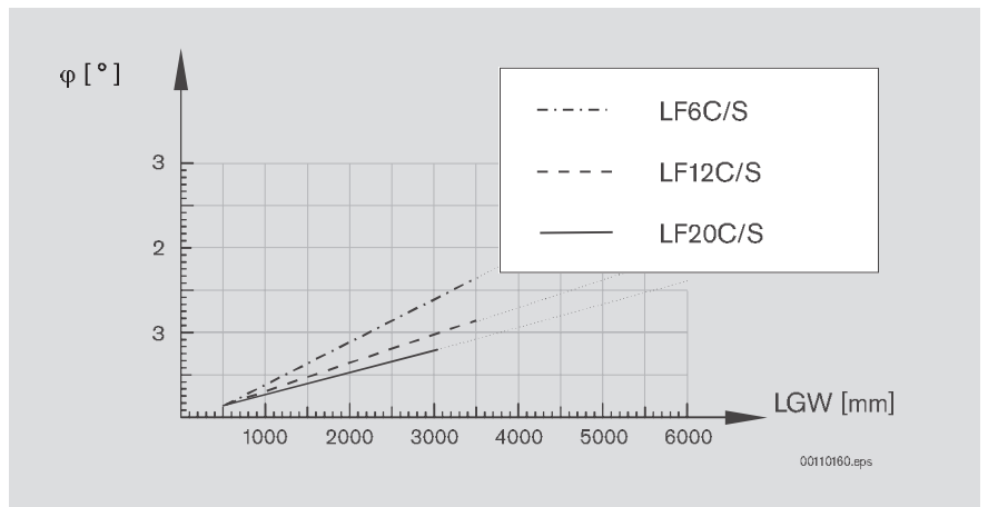
Diagrama 5: Ángulo de torsión
