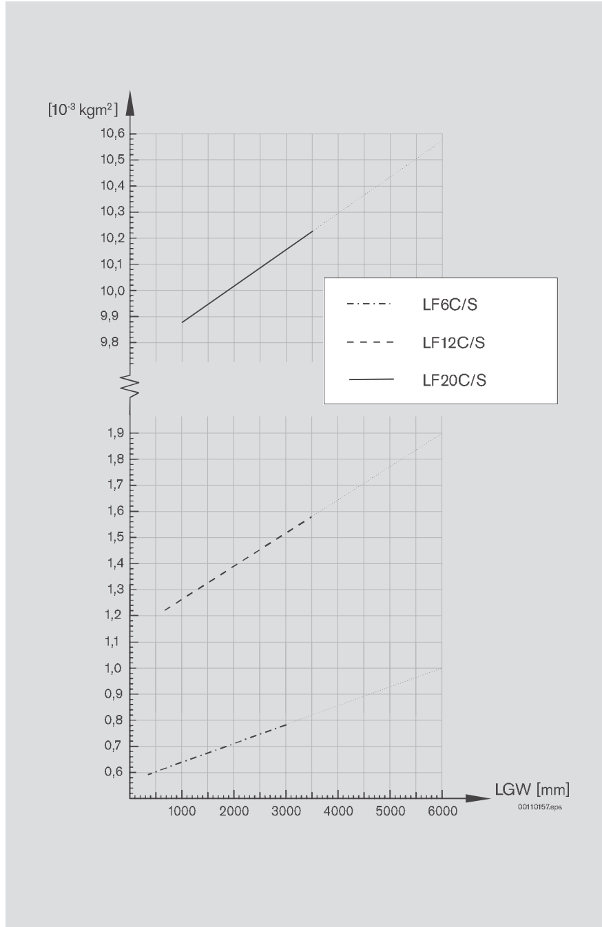
Diagrama 2: Inercia
