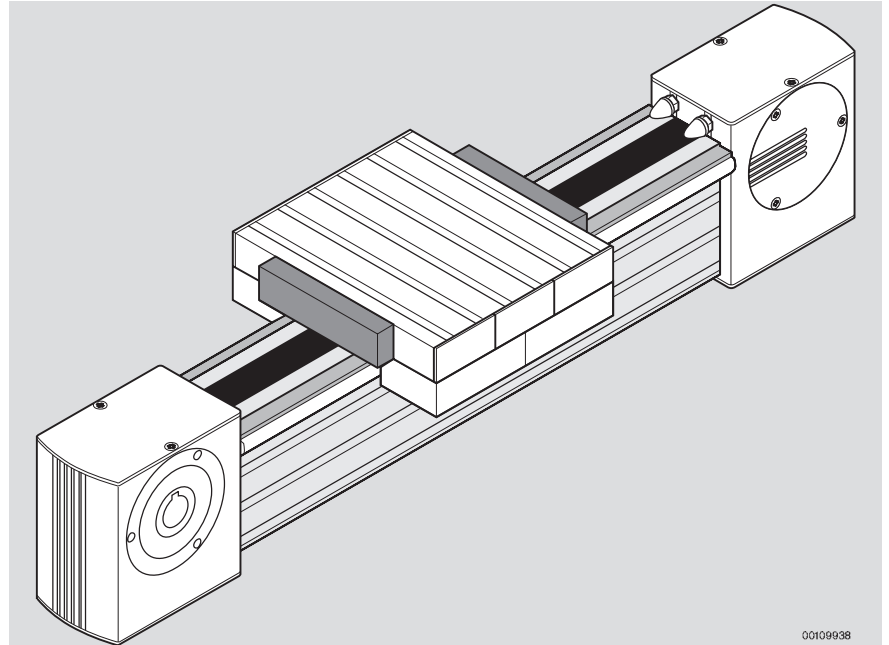
Eje completo LF20C
