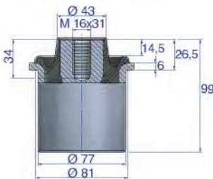
CONO HIDRÁULICO 31
