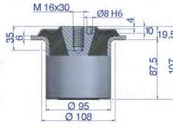
CONO HIDRÁULICO 70
