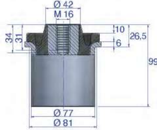
CONO HIDRÁULICO 32
