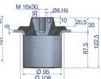
CONO HIDRÁULICO 71
