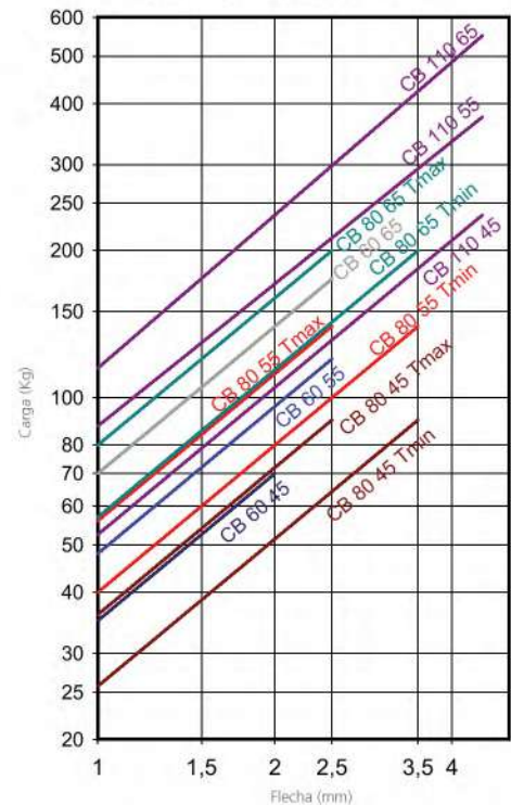
CURVAS DE CARGA FLECHA AMC AMC-MECANOCAUCHO® TIPO CB
