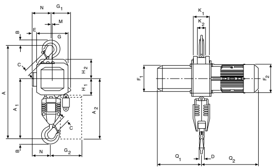
Modelo CPE/CPEF con gancho de suspensi3n, 3.200 - 5.000kg, dos ramales
