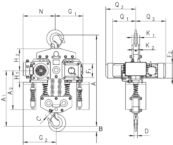
Modelo CPE/CPEF 100-2 con gancho de suspensi3n, 10.000kg
