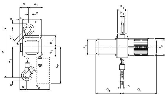
Modelo CPE/CPEF con gancho de suspensi3n, 1.600 - 3.000kg, un ramal
