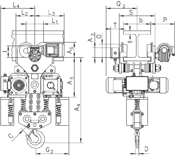
Modelo CPE/CPEF con carro eléctrico integrado, 10.000 kg
