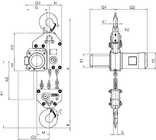
Modelo CPE/CPEF 75-1,6 con gancho de suspensi3n, 7.500kg
