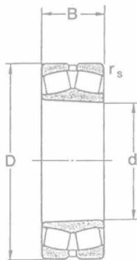
Alésage conique 1/12
