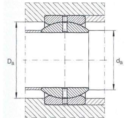
GE..ZO - Medidas de montaje
