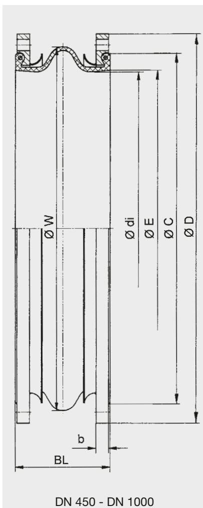
Tipo A-1 Compensador universal, sin arriostramiento
